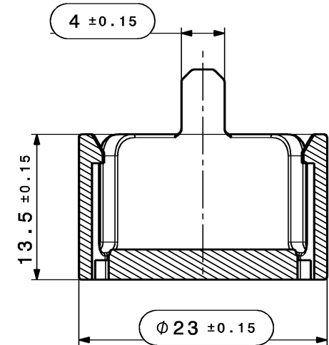
Schnitt A-A CUT A-A
