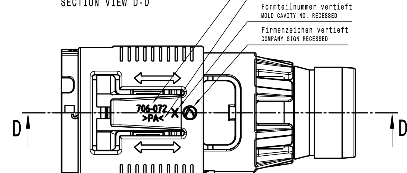
Schnittansicht D-D SECTION VIEW D-D
