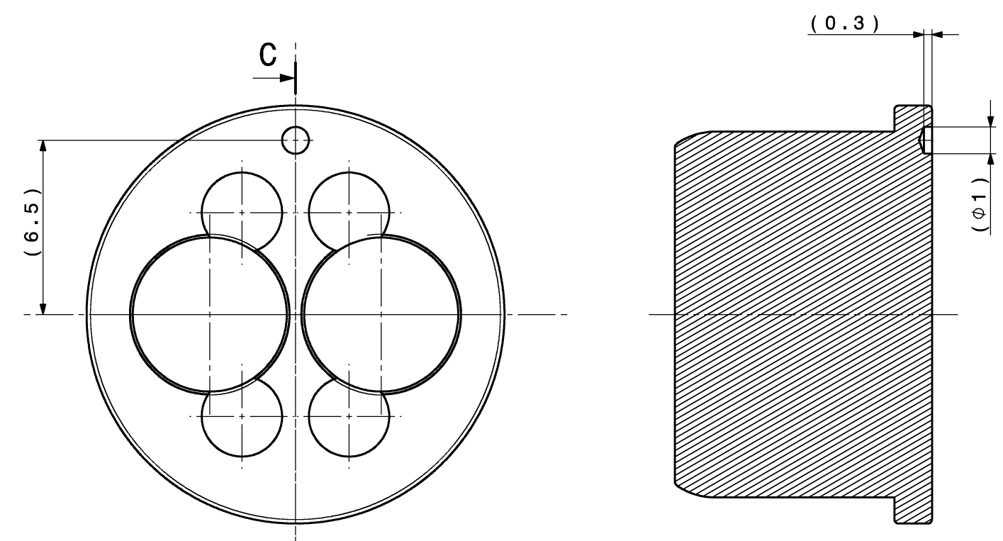
Schnittansicht C-C Maßstab: 5:1 SECTION-CUT C-C SCALE: 5:1
